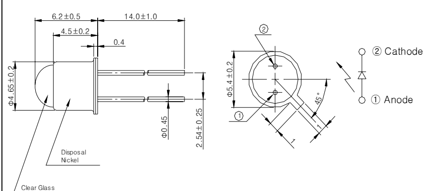
■ DIMENSIONS (Unit:mm)
