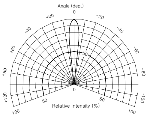
■ Radiant Pattern
