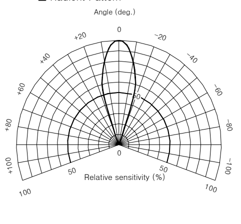
■ Radiant Pattern
