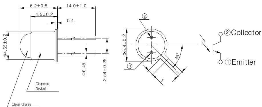
■ Dimensions (mm)
