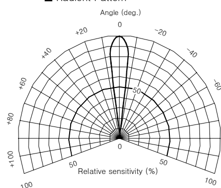
■ Radiant Pattern
