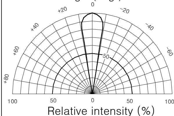
■ Radiant Pattern
